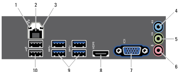
Rysunek 2. Widok na panel tylny
